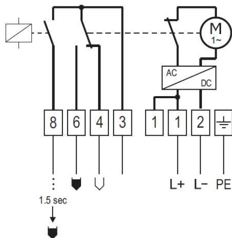
Схема электрического подключения для сигнализатора с напряжением питания от источника постоянного тока с опцией D4
