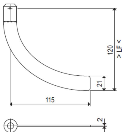
Измерительная лопасть M8V, укрепленная, для очень малых присоединений
