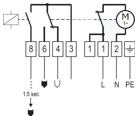
Схема электрического подключения для сигнализатора с напряжением питания от источника переменного тока с опцией D4
